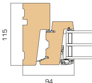
2 Vandret snit i sidekarm
