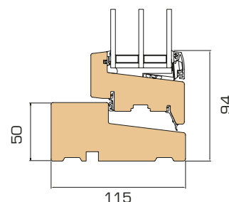
3 Lodret snit i bundkarm
