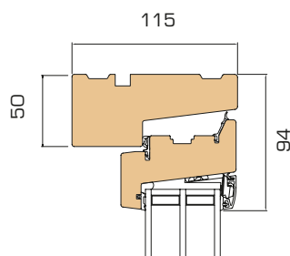
1 Lodret snit i overkarm/ramme
