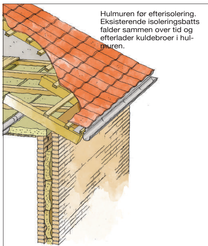
Isoleringsmaterialet indblæses i hulmuren med et specielt mundstykke som sikrer, at hulmuren isoleres effektivt. Efter isolering udfyldes hullerne i ydermurens fuger igen, så indgrebet ikke kan ses.
